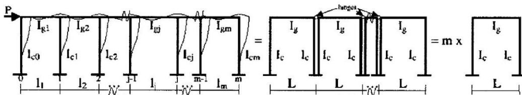
شکل ۱۰- روش پیشنهادی حسینی و ایماق ناینبیری برای محاسبه سختی طبقات [۲۰]
