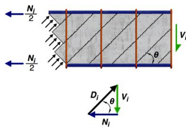
شکل ۸-۱۱ ب تجزیه نیروی برشی V_i به نیروی فشاری قطری D_i و نیروی کششی محوری N_i در یک دیوار لوله
