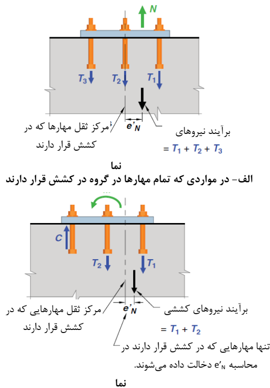
شکل ۶-۱۸ تعریف e'_N برای گروه مهار
