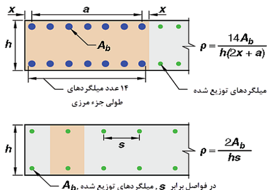
شکل ۲۰-۱۹ نسبت آرماتور طولی برای جز مرزی در یک دیوار سازه‌ای عادی
