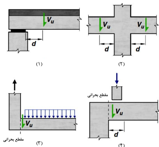
شکل ۲-۱۱-۲-۱۱-پ شرایط معمول تکیه‌گاه تیر برای وارد کردن بار و محل مقطع بحرانی
