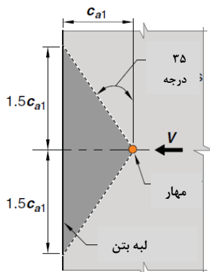
پلان ب- شکست مخروطی بتن در برش
