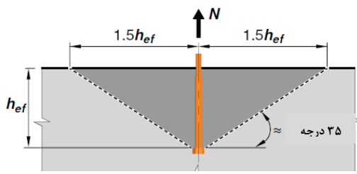
نما الف- شکست مخروطی بتن در کشش
