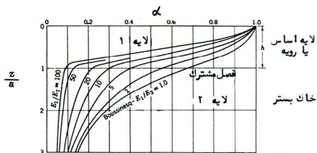
شکل ۸-۵- منحنی های تاثیر برمستتر برای محاسبه تنش فشاری قائم
