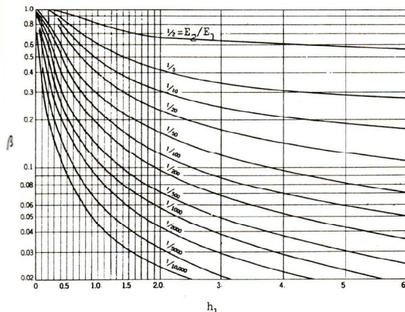
شکل ۸-۶ - برمیستر برای محاسبه افت و خیز حداکثر
