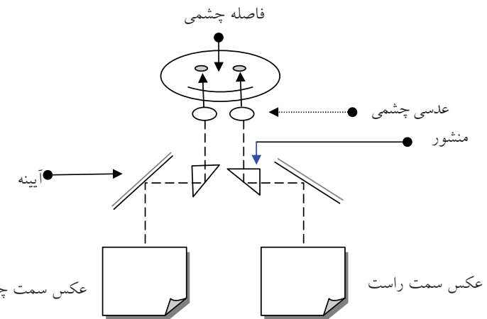
شکل ۱-۳۳: اساس دستگاه استریوسکوپ آینه‌دار
