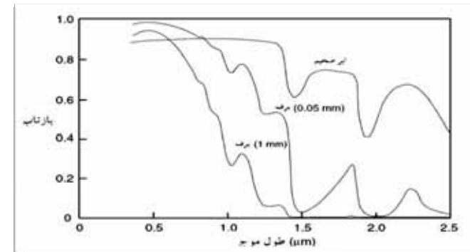
شکل ۱-۵: منحنی بازتاب طیفی برف و ابر (Rees 2006)
