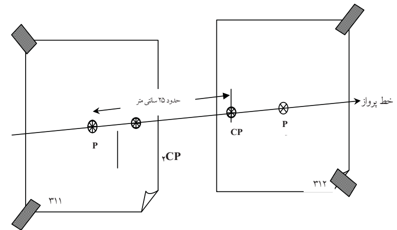
شکل ۱-۴۱: جفت عکس متوالی هوایی آماده شده به منظور برجسته‌بینی با استریوسکوپ آئینه‌دار
