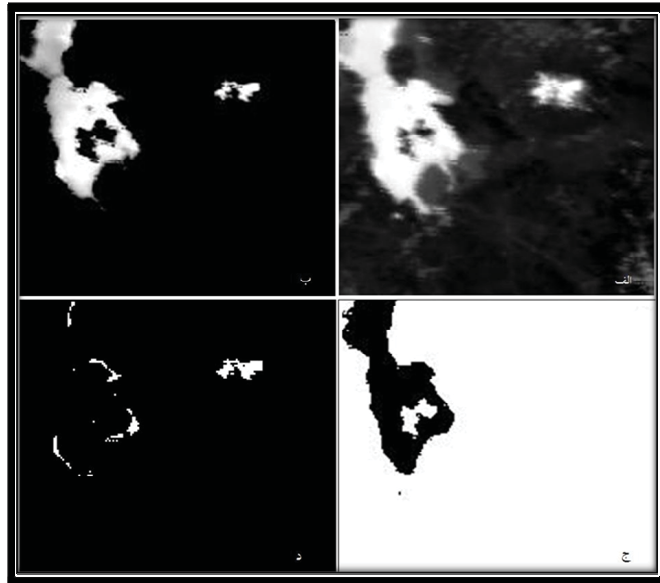
شکل ۲-۵: تصویر حاصل از: الف) NDSI، ب) NDSI > 0.4 ، ج) p_2 > 0.11 و د) آشکارسازی برف براساس شاخص NDSI و آستانه‌های تعریف شده
