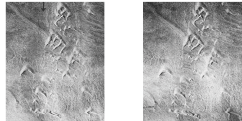
شکل ۳-۲۲: استریوگرامی از بارخان‌ها
