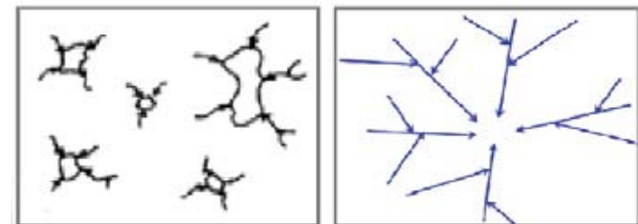
شکل ۳-۶: شبکه زهکشی همگرا: در این الگو انشعابات آبراهه‌ها از اطراف به نقطه مرکزی جریان می‌یابند و معمولاً در چاله‌های بزرگ که ممکن است منشاهای متفاوت مانند فرسایشی در حوضه‌های آهکی، تکتونیکی و آتشفشانی (کالدر، دهانه‌های بزرگ) باشند به وجود می‌آیند.
