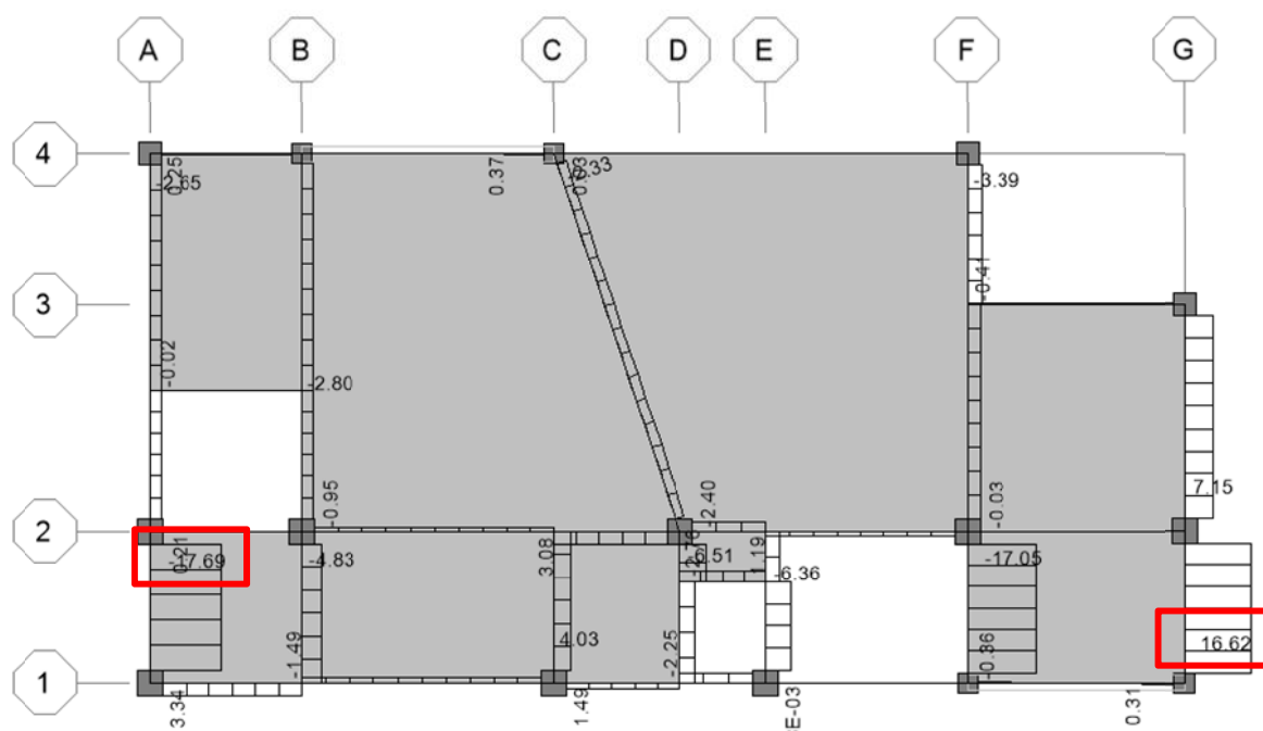
شکل (37): برش اعضای انتخاب شده ناشی از تحلیل سازه
