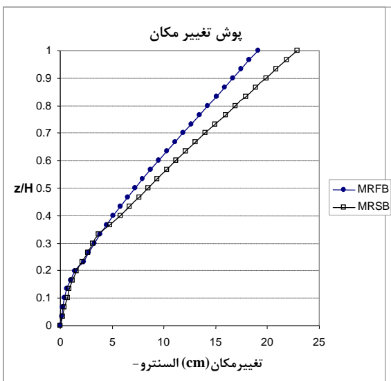
الف. پوش تغییر شکل برای مدل های با مخزن المان محدود ب. پوش تغییر شکل برای مدل های با مخزن جرم افزوده شکل ۱۳- اثرات مدل سازی سنگ پی بر پوش تغییر شکل - زلزله السنترو
