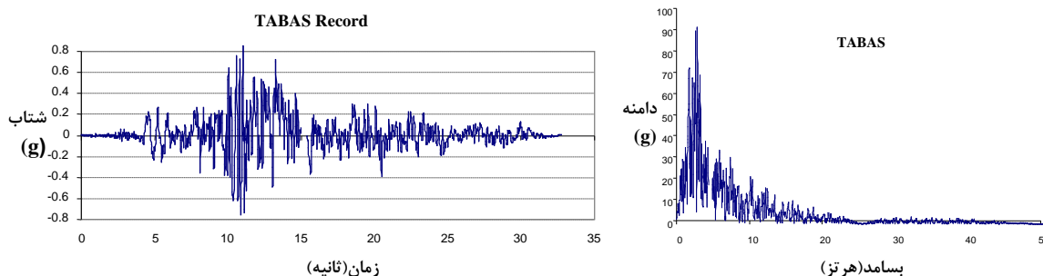
شکل ۵- نمودار محتوای فرکانسی (راست) و شتاب نگاشت (چپ) زلزله طیس [۱۸]
