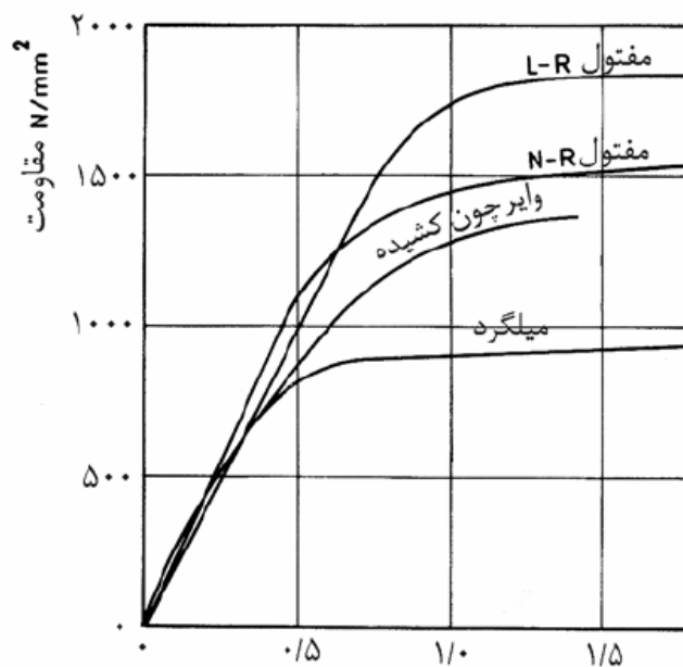
شکل ۲-۱۰ منحنی های تنش - کرنش برای فولاد پیش تنیدگی
