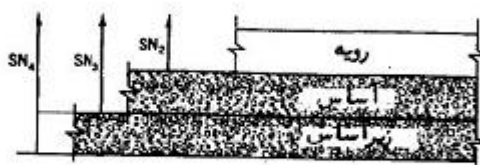
شکل ۴ روش وین تیل برای تعیین حداقل ضخامت لایه‌های روسازی
