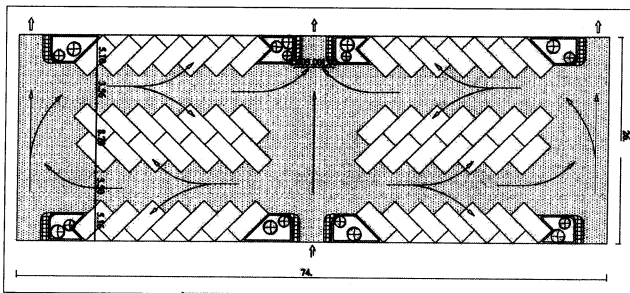
شکل ۵-۱۱: الگوی پارکینگ ۴۵ درجه خودروهای سواری
