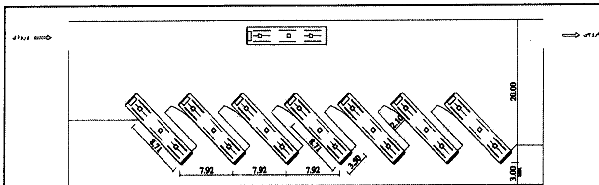
شکل ۵-۱۵: الگوی سکوی زاویه‌دار با زاویه ۴۵ درجه
