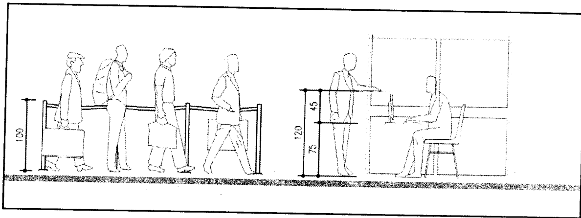
شکل ۶-۲: غرفه فروش بلیت
