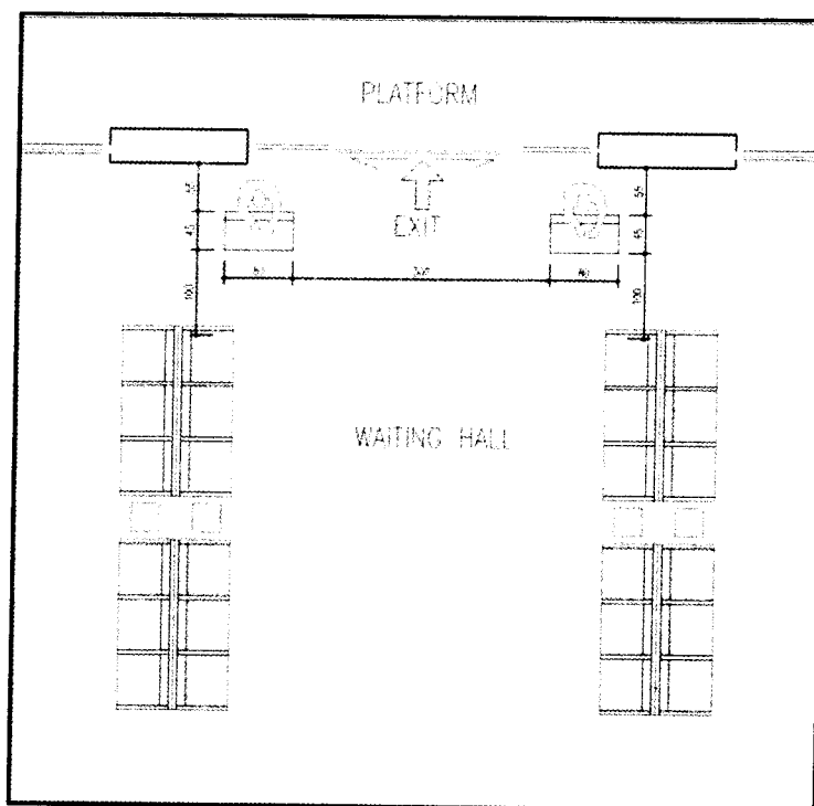
شکل ۳-۶: سالن انتظار و دروازه خروجی
